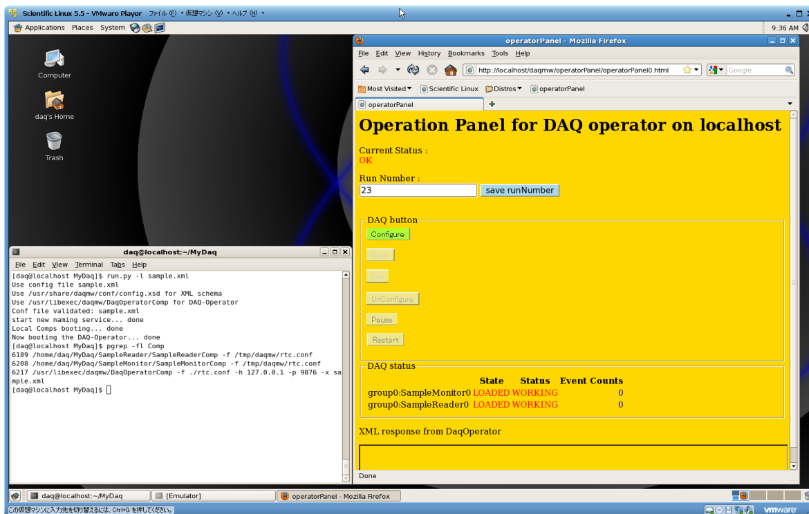
図 11 WebUI。エミュレータを動かし(下のパネルに納められている Emulator と書かれた端末で起動している)、 run.py -l sample.xml として各コンポーネントを起動し、Web ブラウザで http://localhost/daqmw/operatorPanel/operatorPanel10.html にアクセスしたところ。
