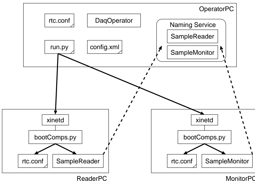
図 15 リモートブートのしくみ。
